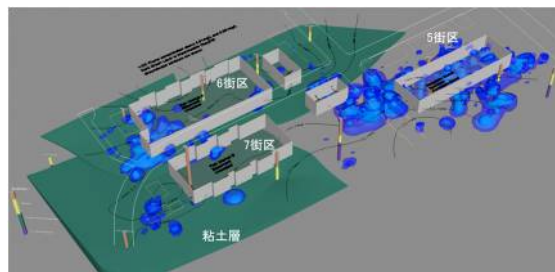
図2 粘土層（緑色）と汚染との関係 5街区の下には粘土層（遮水層）がないので深くまで汚染が広がっていたようです
