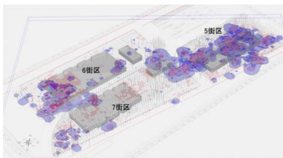
図3 土壌汚染の浄化を行った箇所メッシュ(10m四方)が、赤い色で塗られている個所で土壌浄化工事が行われています。
